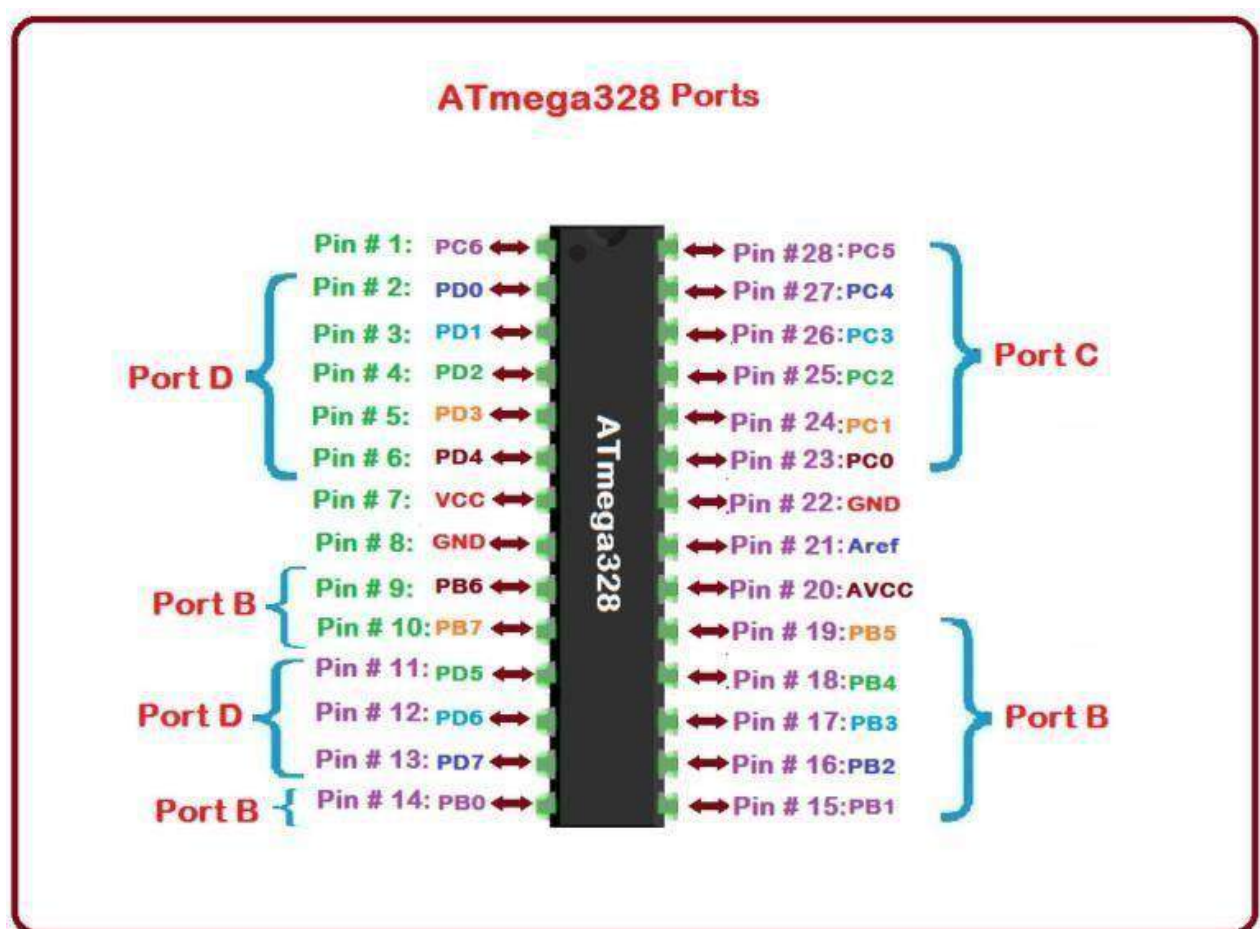
Fig 2 ATmega 328 port
